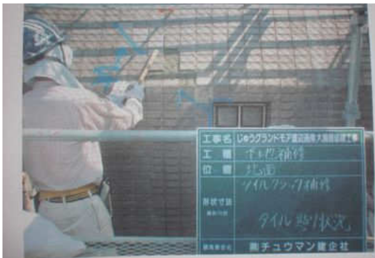
タイル張替え工法
