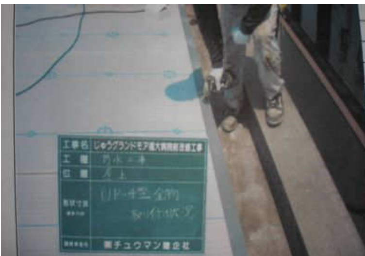
塩ビシート露出機械固定工法
